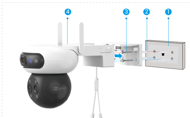
Fig. 2 Väggmontering
